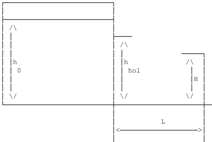
Рис. ПЗ.1. Схема для расчета истечения жидкости из отверстия в резервуаре
